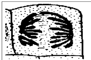
Рис. 4. Схема анафазі
