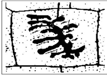
Рис. 3. Схема метафазі
