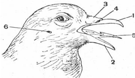
Рис. 69. Голова голуба:
