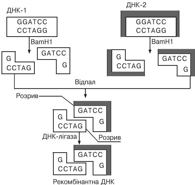
Рис. 5.1. Схема конструювання рекомбінантної ДНК (за Хопевудом Д., 1984)
