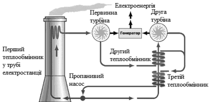
Рисунок 3.31 – Схема типової теплової електростанції
