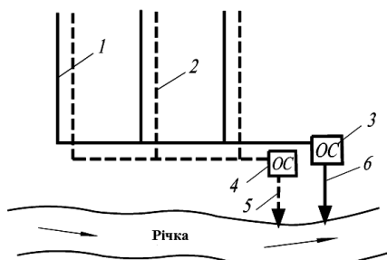
Рисунок 3.7 – Повна роздільна система водовідведення
