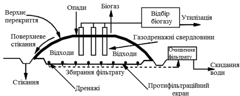
Рисунок 3.34 – Схема полігона ТПВ
