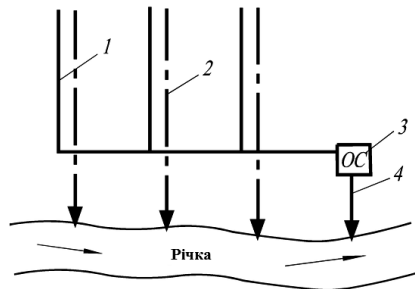
Рисунок 3.8 – Неповна роздільна система водовідведення
