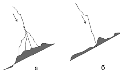
а – дельта; б – естуарій Рисунок 3.1 – Гирлова область річки
