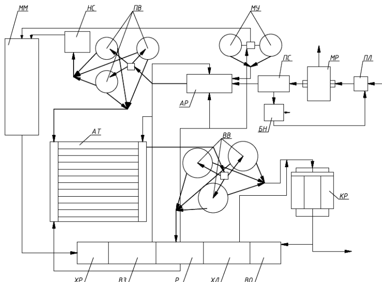
ПЛ – приймальний лоток, МР – механічні решітки, ПС – пісколовловач; АТ – аеротенк, АР – аератор, ПВ – первинний відстійник, НС – насосна станція, ММ – муловий майданчик; КР – контактний резервуар, МУ – мулоуловлювач, Р – резервуар, БН – бункер-накопичувач, ВВ – вторинний відстійник, ХЛ – хлораторна, ХР – хозфікальний резервуар, ВЗ – повітрودувка, ВО – відсік зневоднення осаду Рисунок 3.10 – Міські очисні споруди
