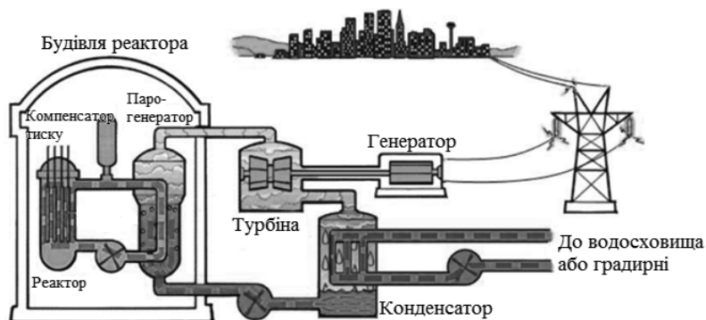
Рисунок 3.32 – Схема роботи АЕС
