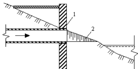
1 – бетонна стінка; 2 – лоток Рисунок 3.14 – Незатоплений береговий випуск
