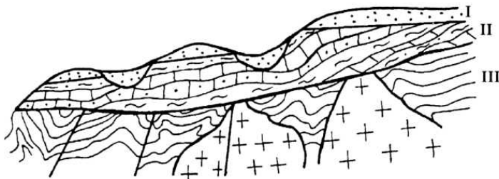
I – шар сучасних відкладень; II – складчаста основа; III – кристалічний фундамент Рисунок 3.40 – Схема геологічної будови території
