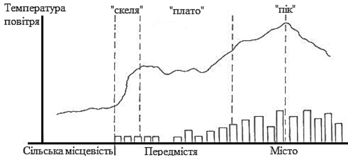
Рисунок 3.26 – Перетин «острова» тепла над містом
