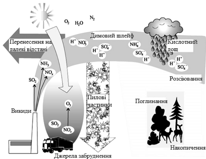
Рисунок 3.23 – Схема розповсюдження забруднень в атмосфері
