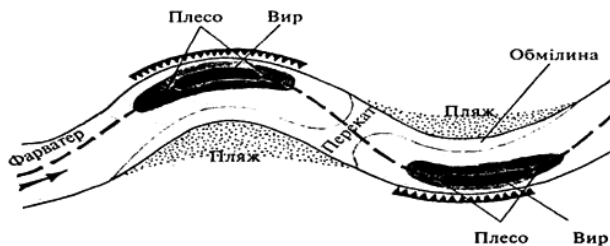
Рисунок 3.17 – Схема руслових форм
