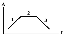
1 – лімітування; 2 – насичення; 3 – пригнічення Рисунок 3.20 – Залежність валової первинної продукції від освітленості
