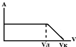
V_l – лімітуюча швидкість потоку; V_k – критична швидкість потоку. Рисунок 3.22 – Залежність валової первинної продукції від швидкості потоку
