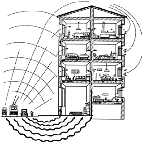
Рисунок 3.28 – Схема розповсюдження шуму у житловому будинку
