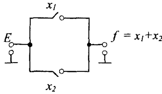
Рис. 2.9. Диз'юнктор у релейному виконанні
