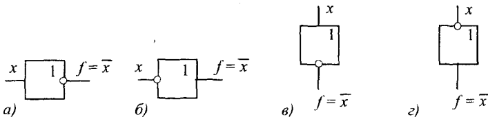
Рис. 2.1 а, б, в, г. Функціональна схема інвертора
