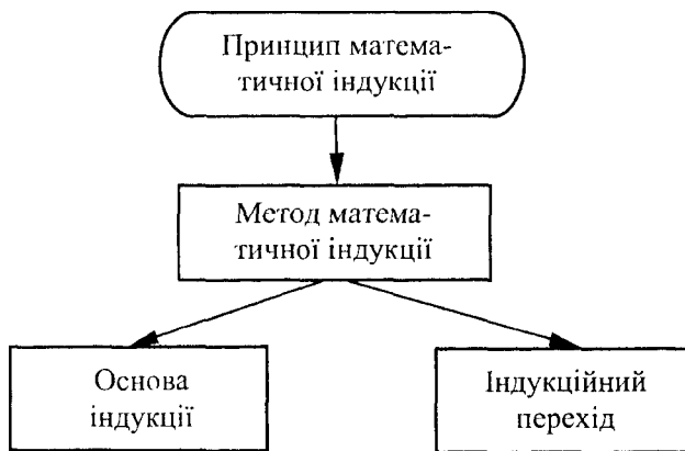
Рис. 1.1. Блок-схема, яка реалізує математичну індукцію
