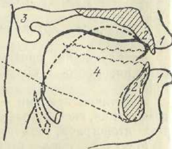
Рис. 6. Зіставна схема рентгенограм приголосних:
