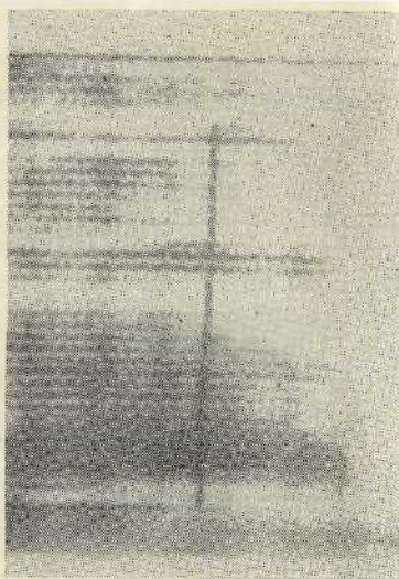
Рис. 14. Положення губ при артикуляції голосного [o].
