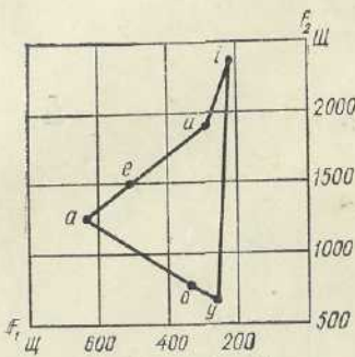
Рис. 30. Класифікаційна схема наголошених голосних, побудована на акустичній основі.
