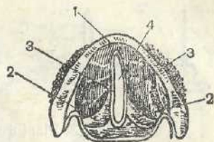
Рис. 2. Поперечний розріз гортані:
