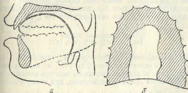
Рис. 34. Схеми рентенограми а і палатограми б приголосних [m'], [θ'] (апикально-альвеолярний різновид).
