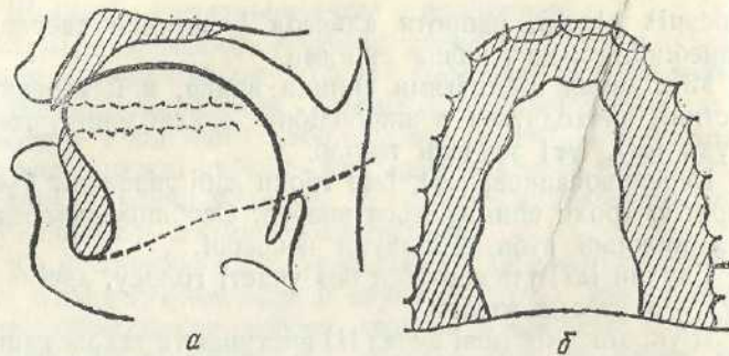
Рис. 40. Схеми рентгенограми а і палатограми б приголосних [ц'], [з'].
