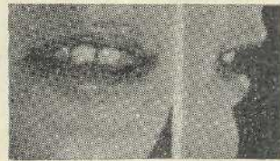
Рис. 26. Положення губ при артикуляції голосного [i].
