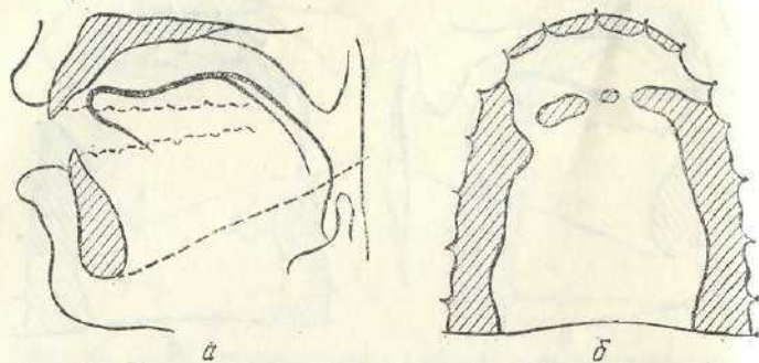
Рис. 51. Схеми рентгенограми а і палатограми б приголосного [r].
