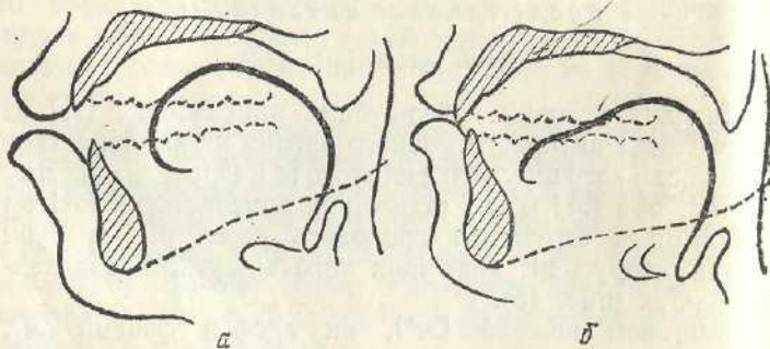
Рис. 46. Схеми рентгенограм: a — губно-губного [w]; б — губно-зубного приголосного [e].
