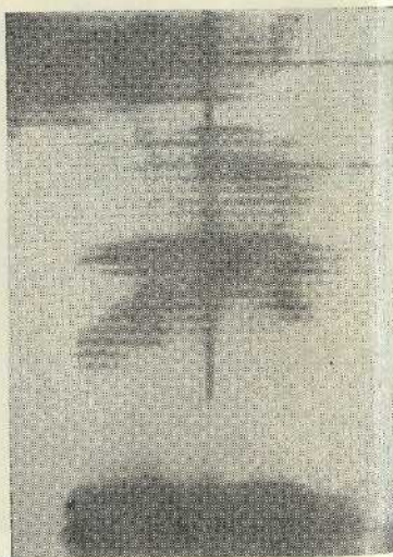
Рис. 24. Спектрограма голосного [u].
