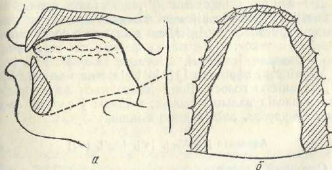
Рис. 39. Схеми рентгенограми а і палатограми б приголосних [ч], [ж].
