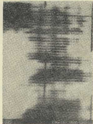
Рис. 20. Положення губ при артикуляції голосного [e].
