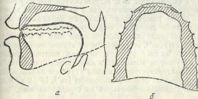
Рис. 33. Схеми рентенограми а і палатограми б приголосних [m], [θ].
