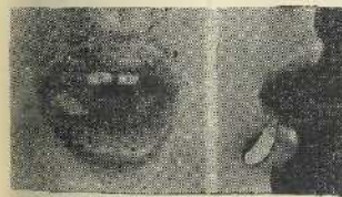
Рис. 20. Положення губ при артикуляції голосного [e].
