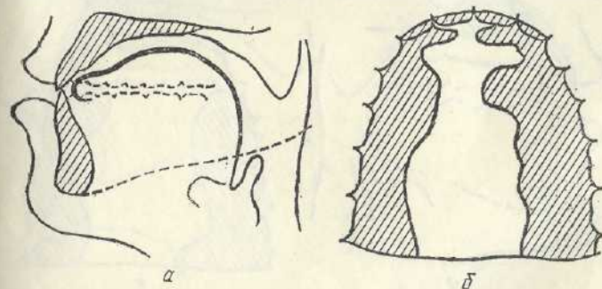
Рис. 37. Схеми рентгенограми a і палатограми б приголосних [c'], [z'].
