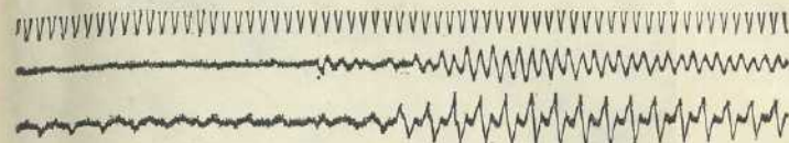
Рис. 7. Осцилограма складу ду в слові дужка.
