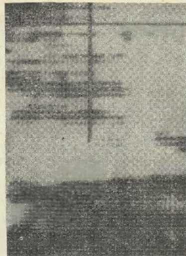
Рис. 15. Спектрограма голосного [o].
