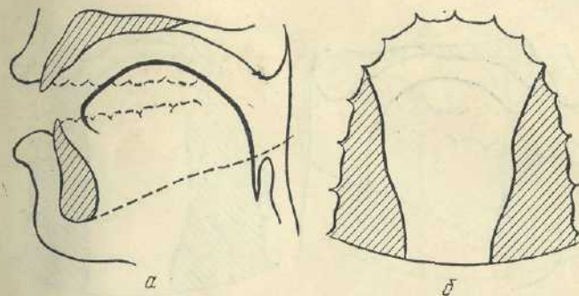
Рис. 19. Схеми рентенограми а та палатограми б голосного [e].
