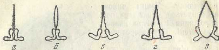
Рис. 3. Різні форми голосової щілини: а — затвір; б — голос; в — шепіт; г — видих; д — вдих.
