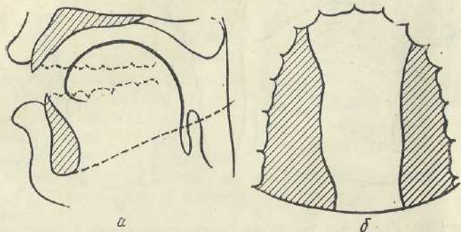
Рис. 22. Схеми рентгенограми a та палатограми b голосного [u].
