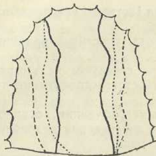
Рис. 5. Зіставна схема палатограм голосних:
