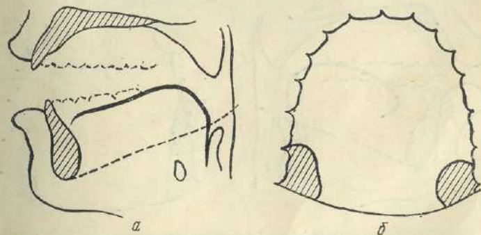
Рис. 10. Схеми рентенограми а та палатограми б голосного [a].
