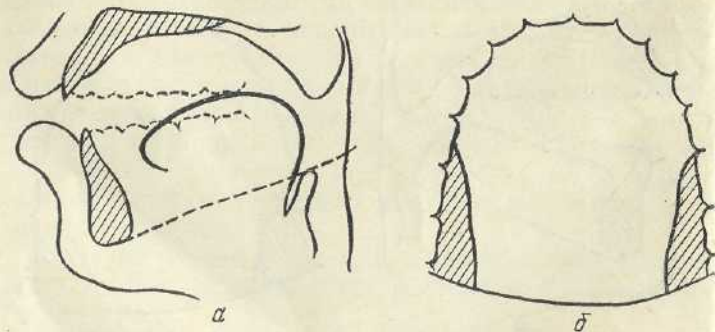
Рис. 13. Схеми рентгенограми а та палатограми б голосного [o].
