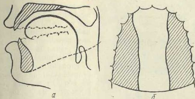
Рис. 25. Схеми рентгенограми a та палатограми b голосного [i].
