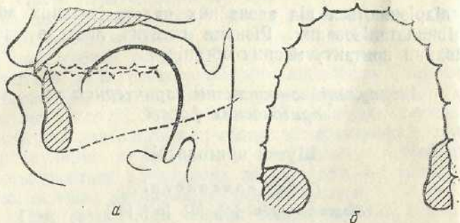
Рис. 32. Схеми рентенограми а і палатограми б приголосного [ʃ].
