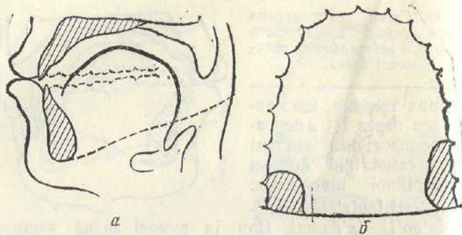
Рис. 45. Схеми рентгенограми a і палатограми б приголосного [м].
