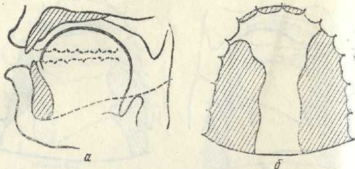
Рис. 53. Схеми рентгенограми a і палатограми b приголосного [j].
