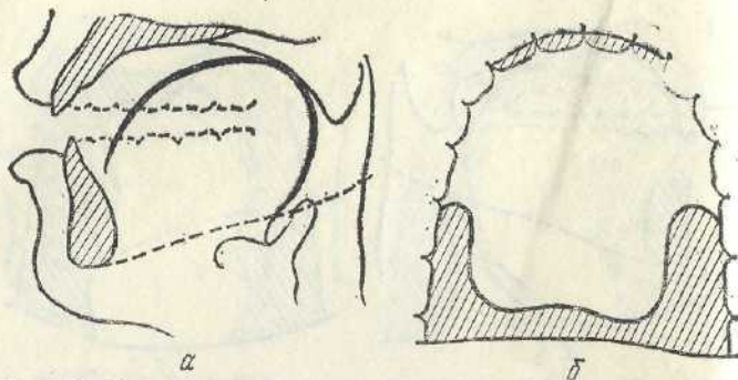
Рис. 42. Схеми рентгенограми а і палатограми б приголосного [x].
