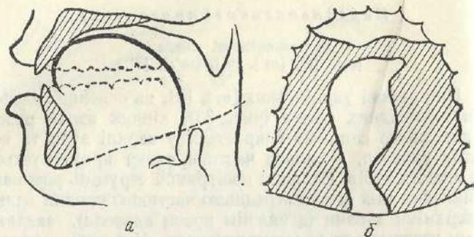
Рис. 35. Схеми рентгенограми a і палатограми б приголосних [m'], [θ'] (дорсально-альвеолярний різновид).
