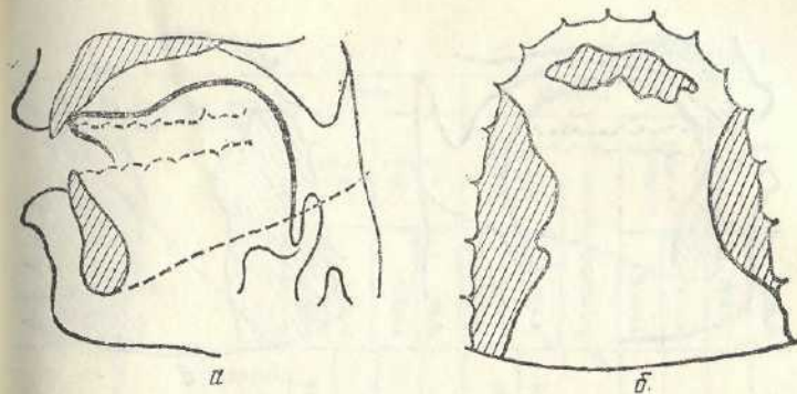
Рис. 52. Схеми рентгенограми а і палатограми б приголосного [r'].
