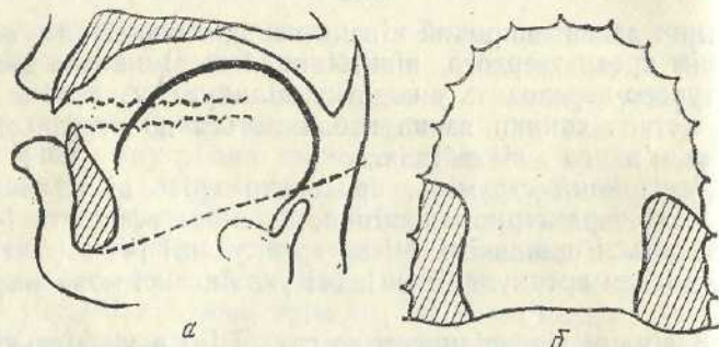
Рис. 43. Схеми рентгенограми а і палатограми б приголосного [x].
