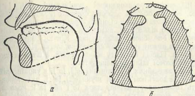
Рис. 36. Схеми рентгенограми a і палатограми б приголосних [c], [z].
