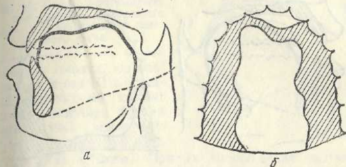
Рис. 41. Схеми рентгенограми а і палатограми б приголосного [ч].
