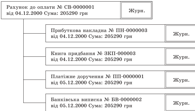
Рис. 7.2. Структура зв'язку документів у програмі "1С: Підприємство" при отриманні ТМЦ і проведенні розрахунків
